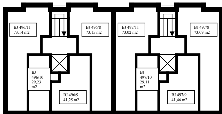
1. nadzemní podlaží
