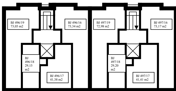
5. nadzemní podlaží
