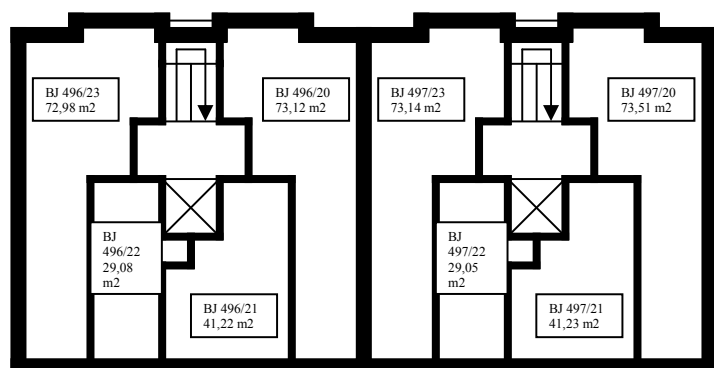
6. nadzemní podlaží
