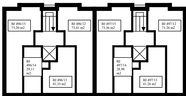
4. nadzemní podlaží
